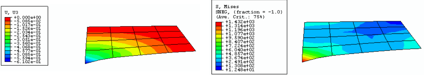
(b) S8R 单元模型位移与应力结果
